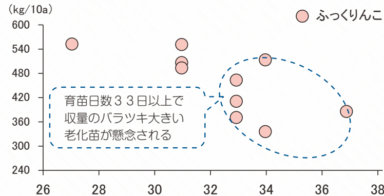
図1 平成30年度 北斗市水稻作況・試験ほの育苗日数と収量の関係
