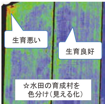
図1 ドローンによるセンシング
