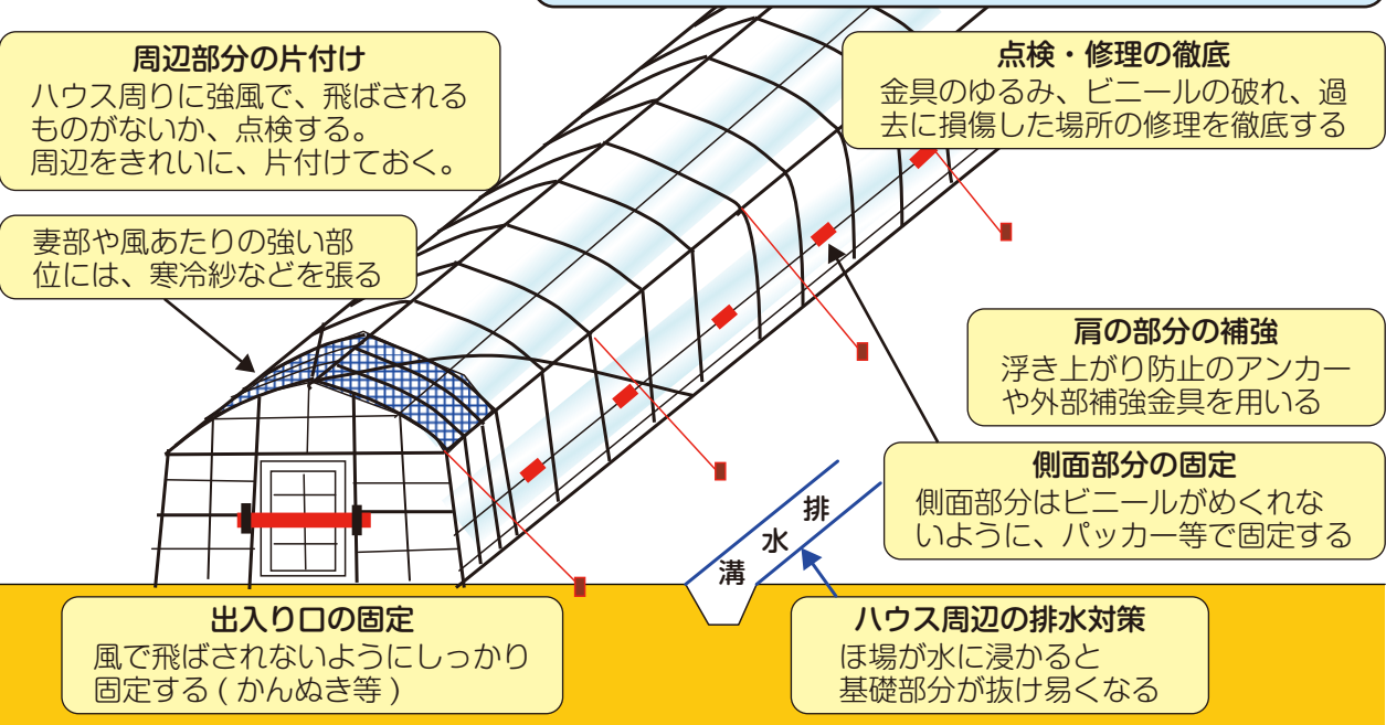
パイプハウスの強化事例
