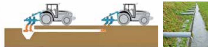
施工断面図1
